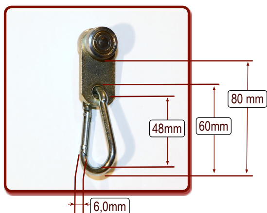
Art.Nr.: 7007met mit Karabinerhaken 6x60mm
