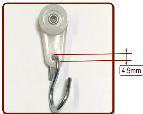
Art.Nr.: 7007bs Anwendungsbeispiel mit offenem S-Haken
