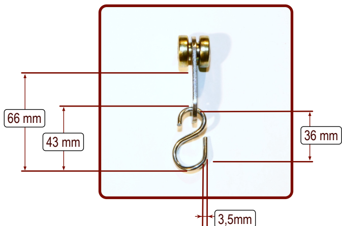
Art.Nr.: 7007mi mit S-Haken
