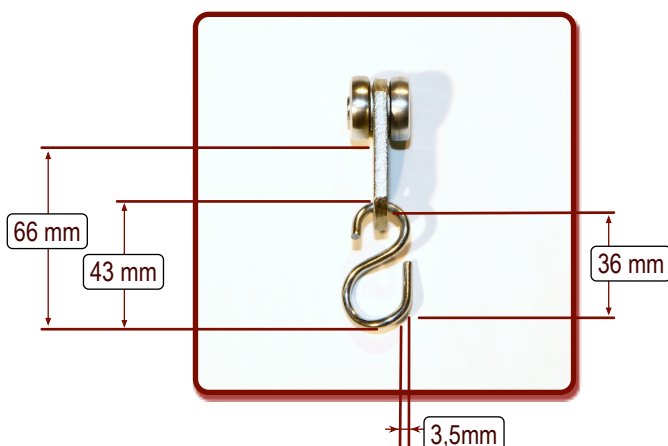
Art.Nr.: 7007met mit S-Haken
