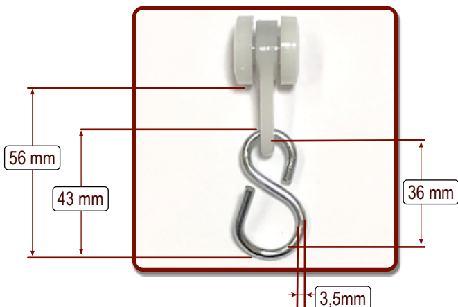
Art.Nr.: 7007bs mit S-Haken
