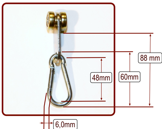
Art.Nr.: 7007mi mit Karabinerhaken 6x60mm
