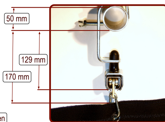
Art.Nr.: 7007met in Track-100 Schiene im G-Haken
