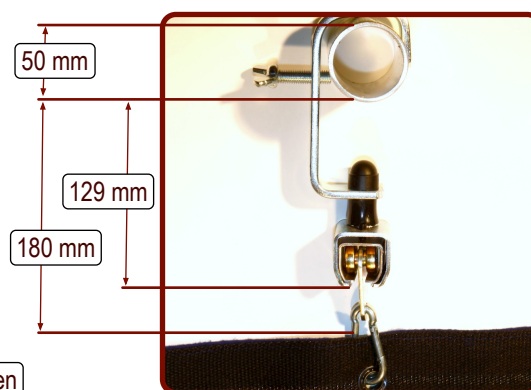
Art.Nr.: 7007mi in Track-100 Schiene im G-Haken
