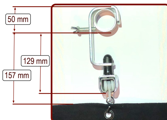
Art.Nr.: 7007bs in Track-100 Schiene im G-Haken
